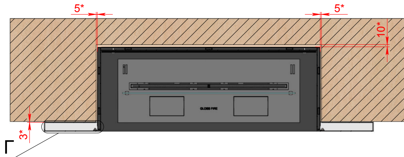
А-А (1 : 10)
