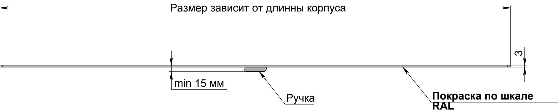
Вид сверху
